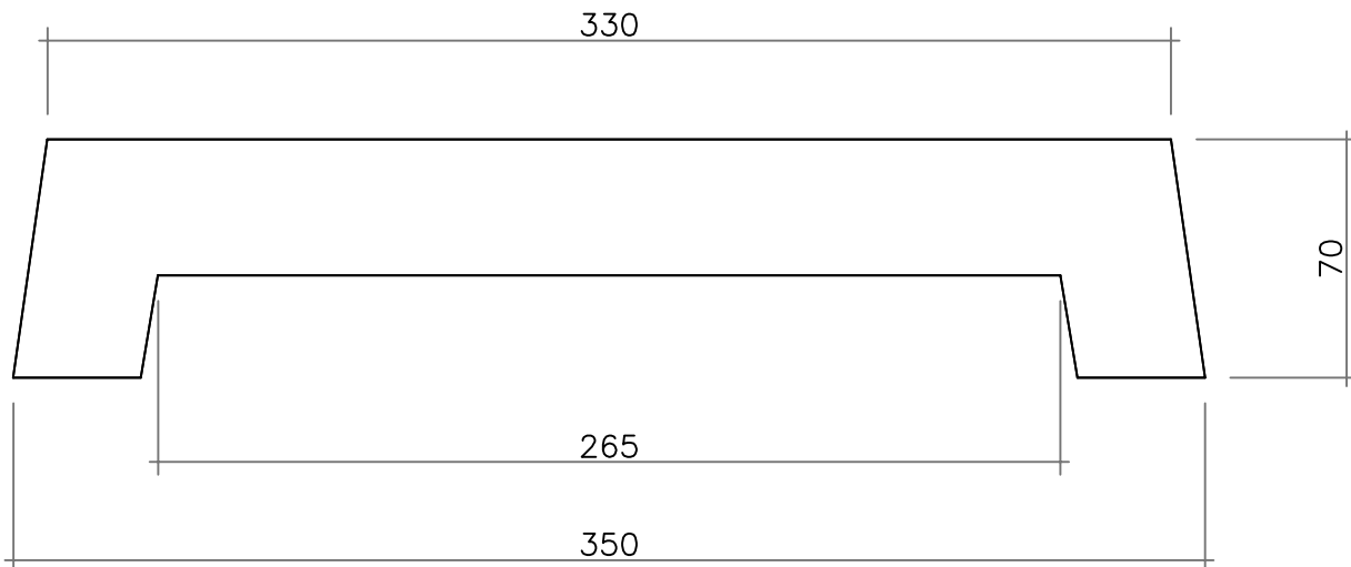
CORTE Sección
